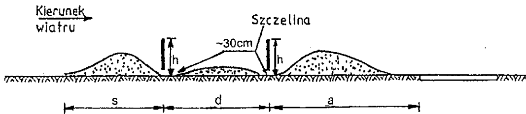
Rys. 7 Ustawienie podwójnych zasłon w terenach o dużych opadach śniegu
