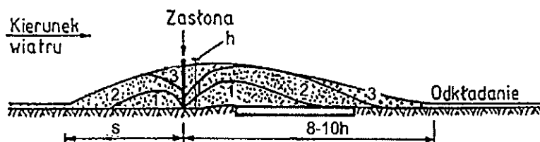
Rys. 6b Powstawanie zasp na drodze zabezpieczonej płotkami lub żywoplotami usytuowanymi niewłaściwie (bez szczeliny dolnej i zbyt blisko drogi)
