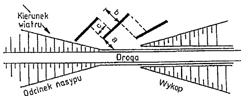
Rys. 13 Zabezpieczenie w przypadku przejścia drogi z nasypu w wykop
